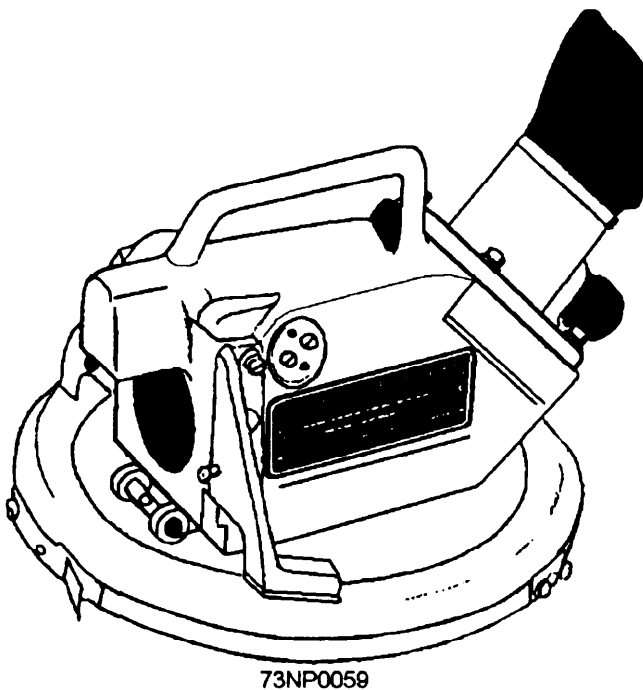
Figure 9-3.—Telescopic alidade.
